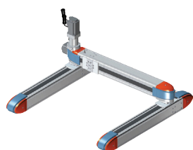
Portale con due assi a cinghia paralleli sormontati da un asse trasversale, serie Elektro Shak Gantry
